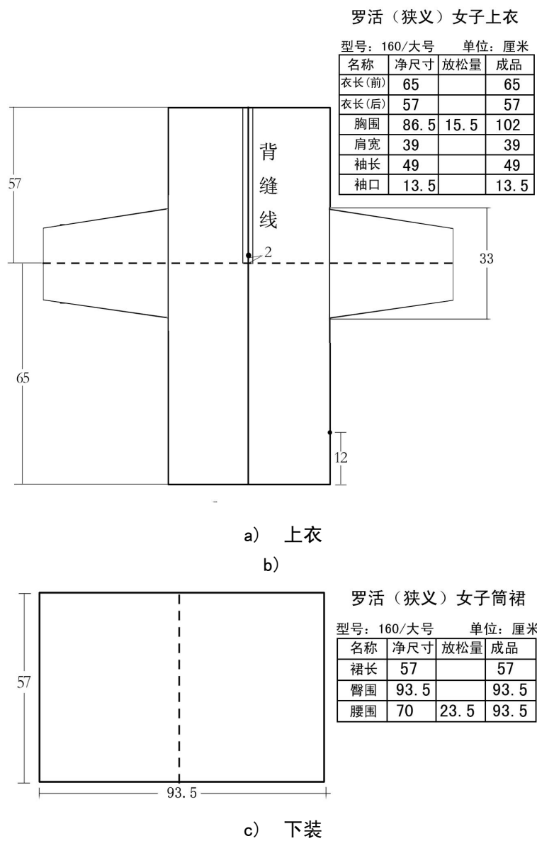
图 B.3 罗活型服装裁剪图
